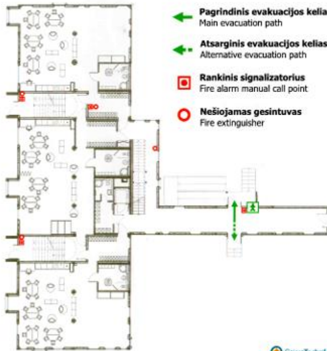
2 pav. modulinio priestato evakavimo planas
